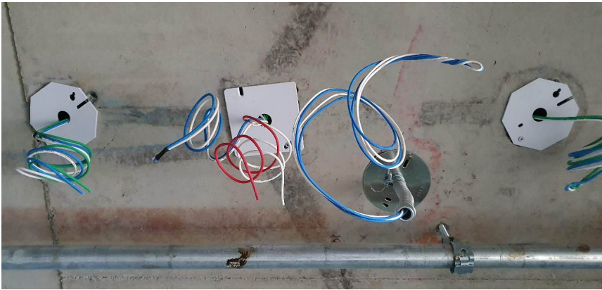
월드평커버 KS 8각, 4각
