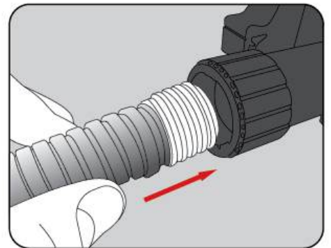
③ 박스 연결
