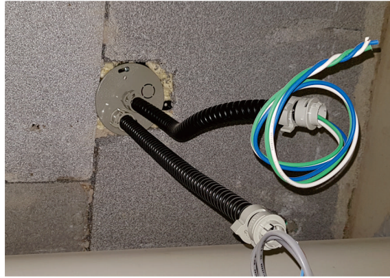
고양향동중흥S클래스 (GWFS 8각2구)
